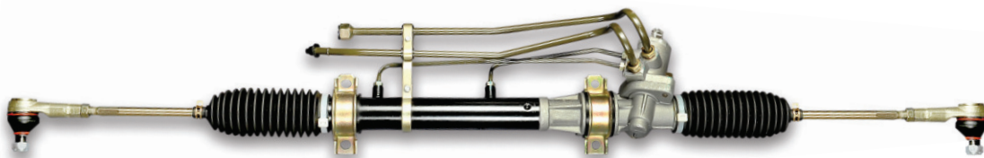
مجموعه جعبه فرمان هیدرولیک پراید/تیا
